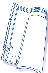
70746 N° 81 - OMÉGA 13 27 x 44,6 cm - 4,2 kg 13 /m 2 Tuilier/ Tile maker Oméga 13 (EDILIANS 69)
