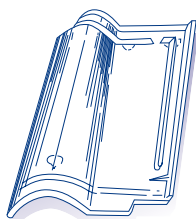
70630 N° 7 bis - ROMANE 27 x 42,5 cm - 4,2 kg 13,2 /m 2 Tuilier/ Tile maker (EDILIANS 31) (MONIER-LAFARGE 13)
